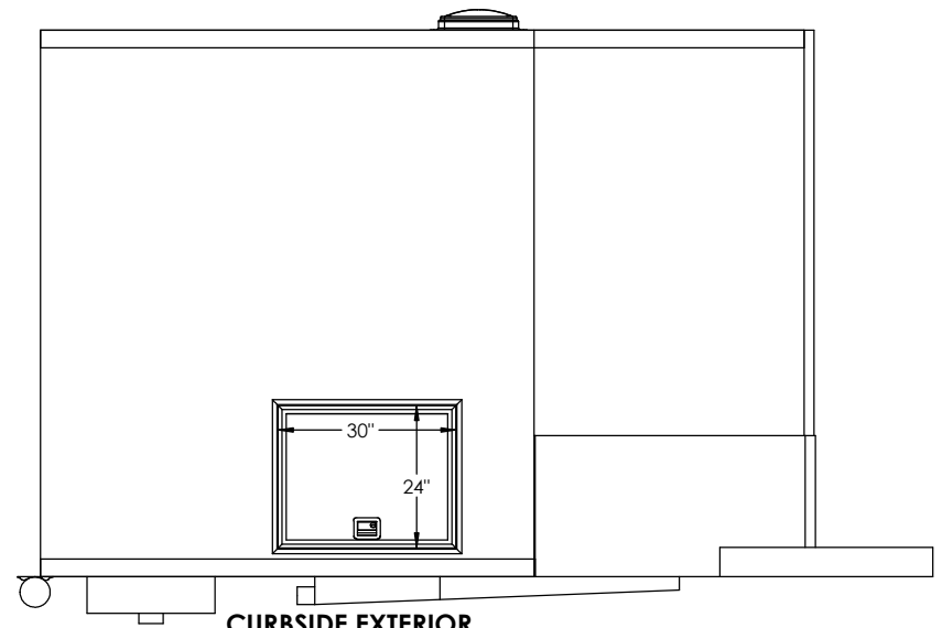
CURBSIDE EXTERIOR
